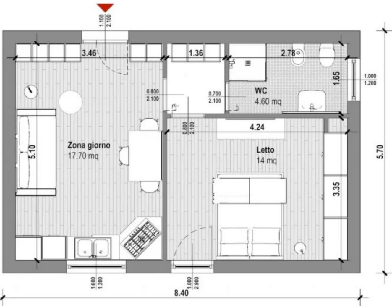
Progetto bilocale da 40 m 2 | Pianta
