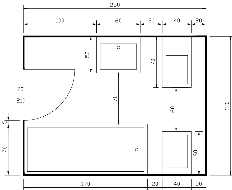
CAMERA DA BAGNO CON DISTRIBUZIONE SANITARI SU DUE PARETI
