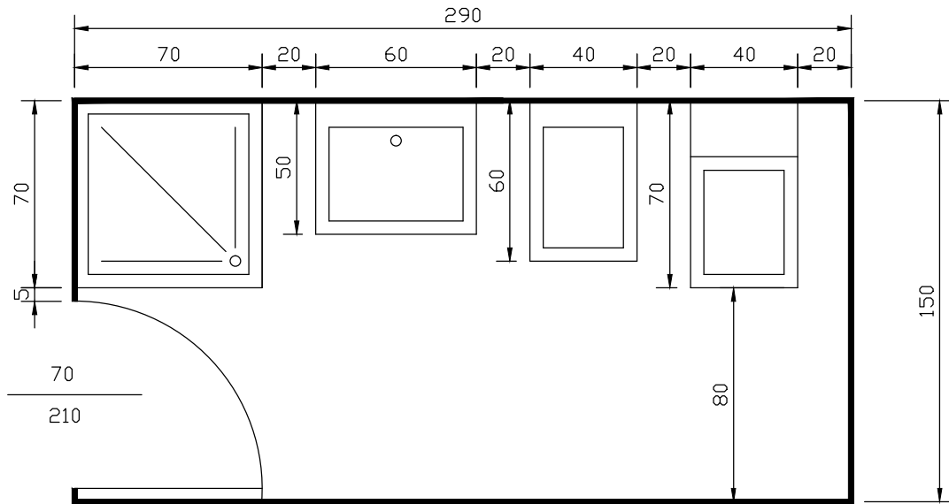
CAMERA DA BAGNO CON DISTRIBUZIONE SANITARI SU UNA PARETE
