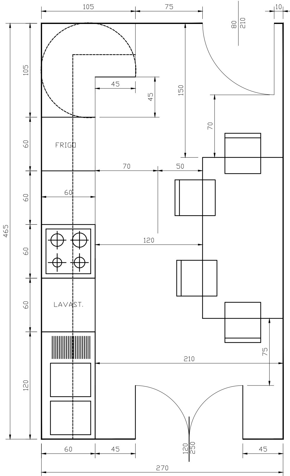
CUCINA CON DISTRIBUZIONE ARREDI SU UNA PARETE
