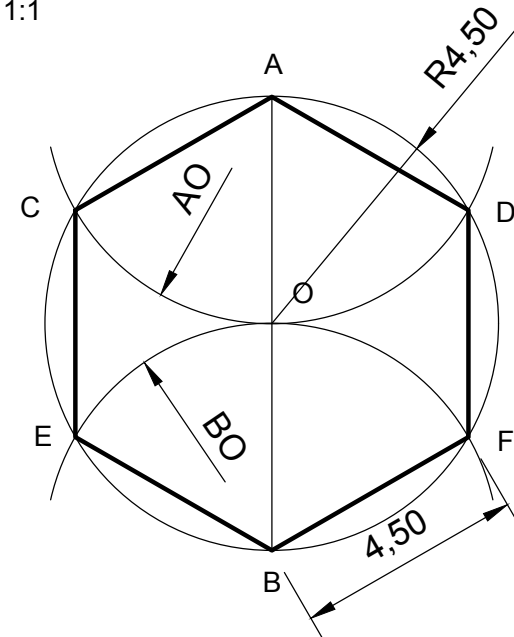
COSTRUZIONE DI UN ESAGONO NOTO IL RAGGIO SCALA 1:1
